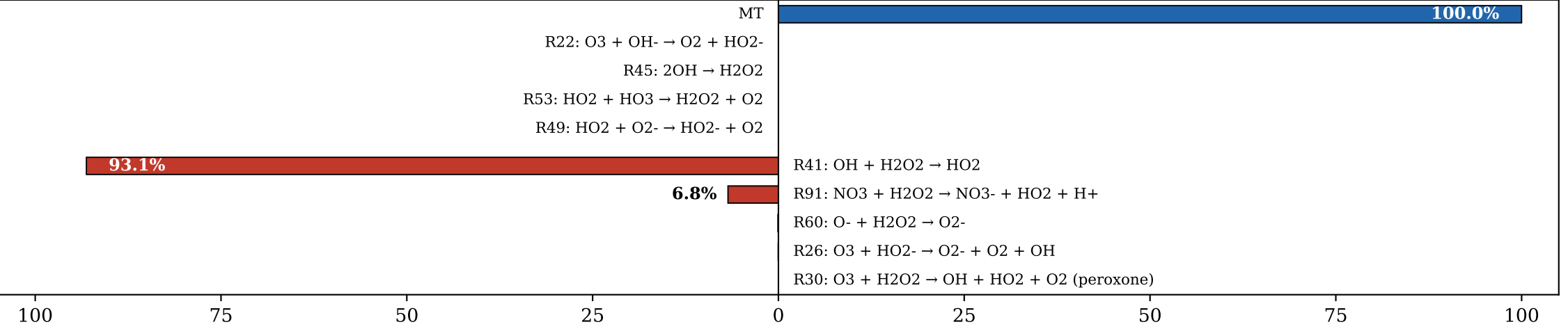
(d) H 2 O 2 (Σsrc = 8.83e-09 M/s)
